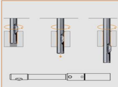
CNC boringontbramer
